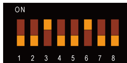
入力選択SW 分圧器
