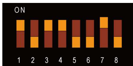
入力選択SW サーミスタ
