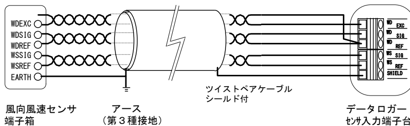
アース(第3種接地)
