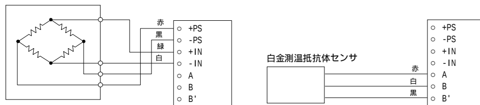
ひずみゲージ式変換器
