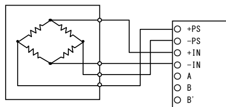
水圧式水位計
